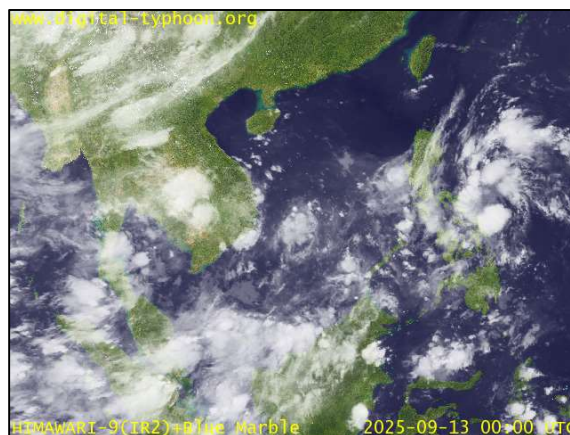
ภาพถ่ายดาวเทียม วันที่ ๑๓ ก.ย. ๒๕๖๘ เวลา ๐๗.๐๐ น.
