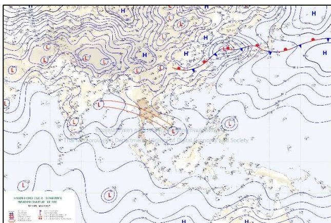
แผนที่อากาศ วันที่ ๑๓ ก.ย. ๒๕๖๘ เวลา ๐๑.๐๐ น.
